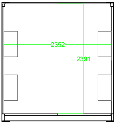
Dwaarsdoorsnede
