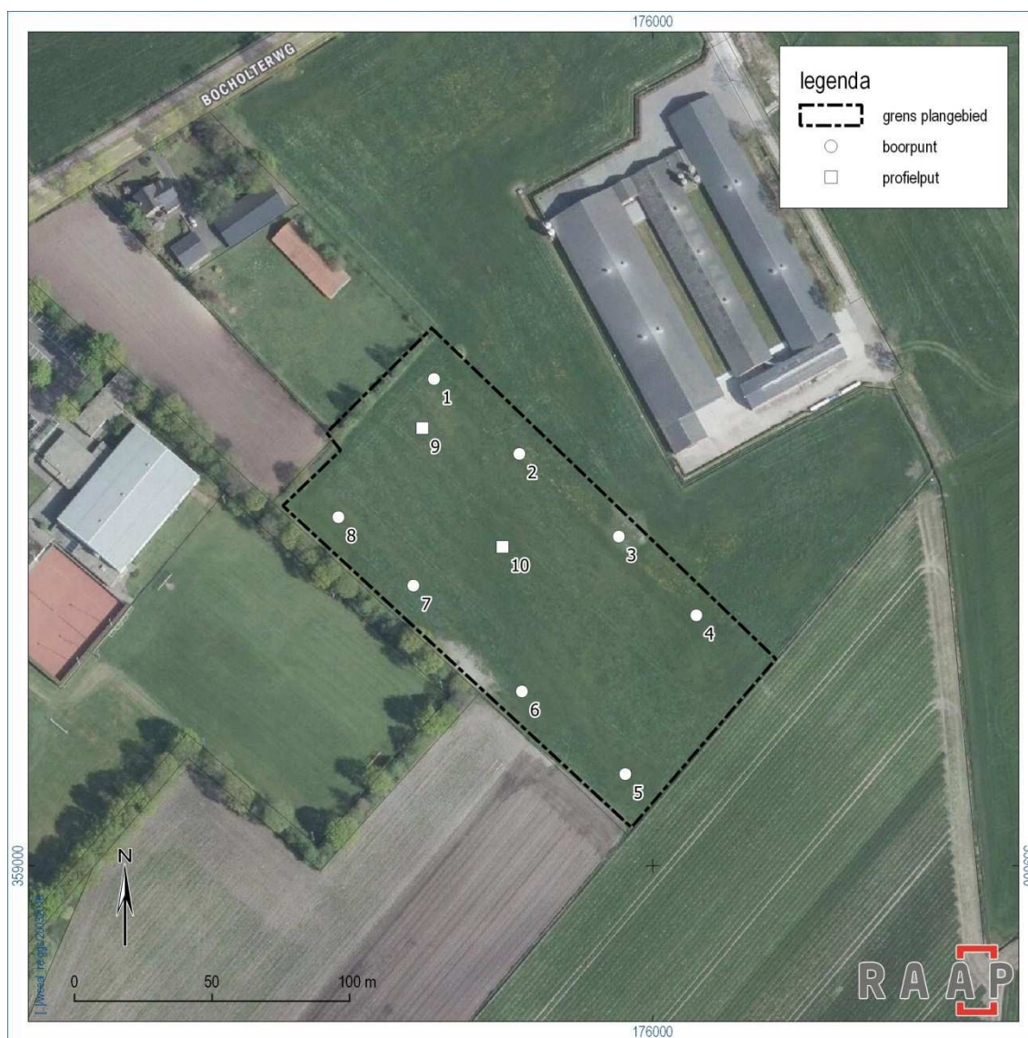
Figuur 9. Boorpuntenkaart.
