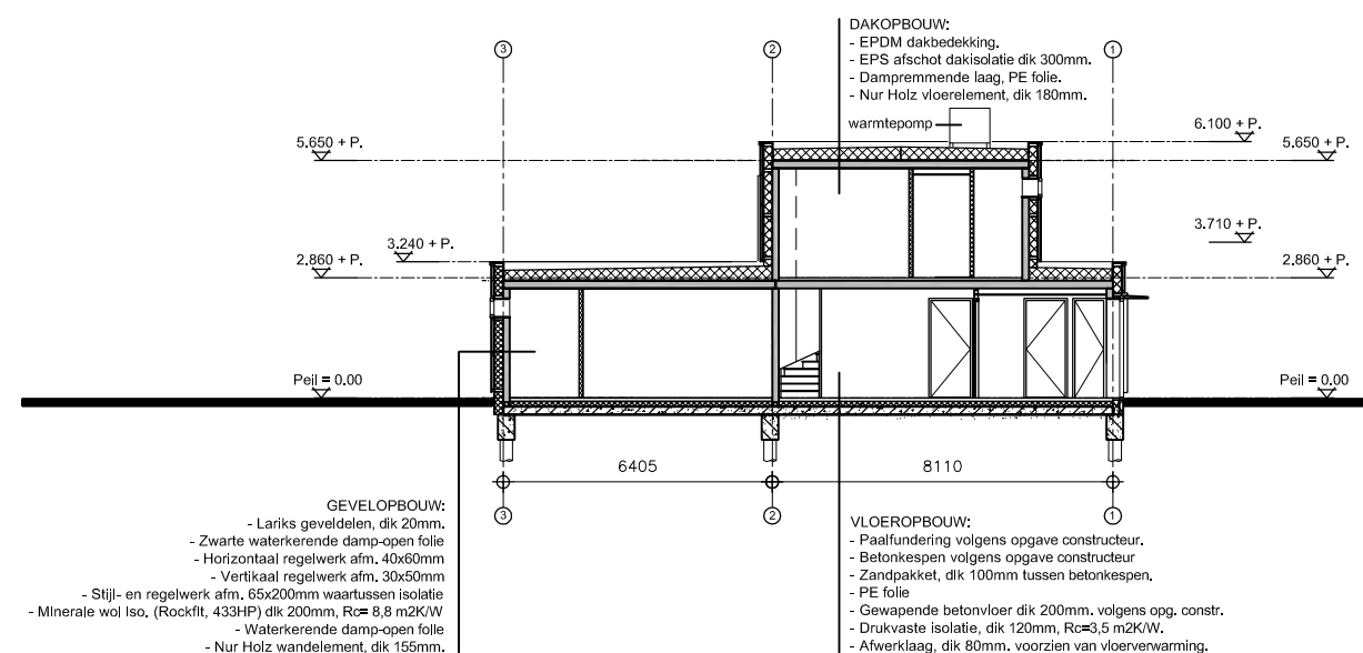
DOORSNEDE B-B
