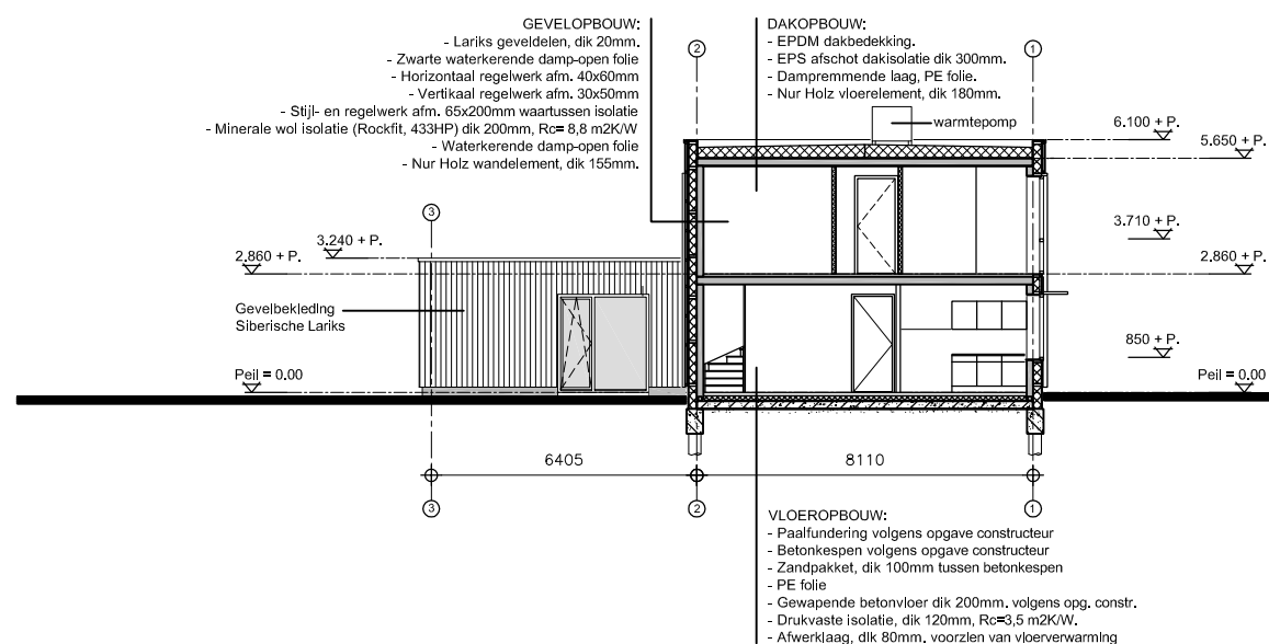
DOORSNEDE A-A
