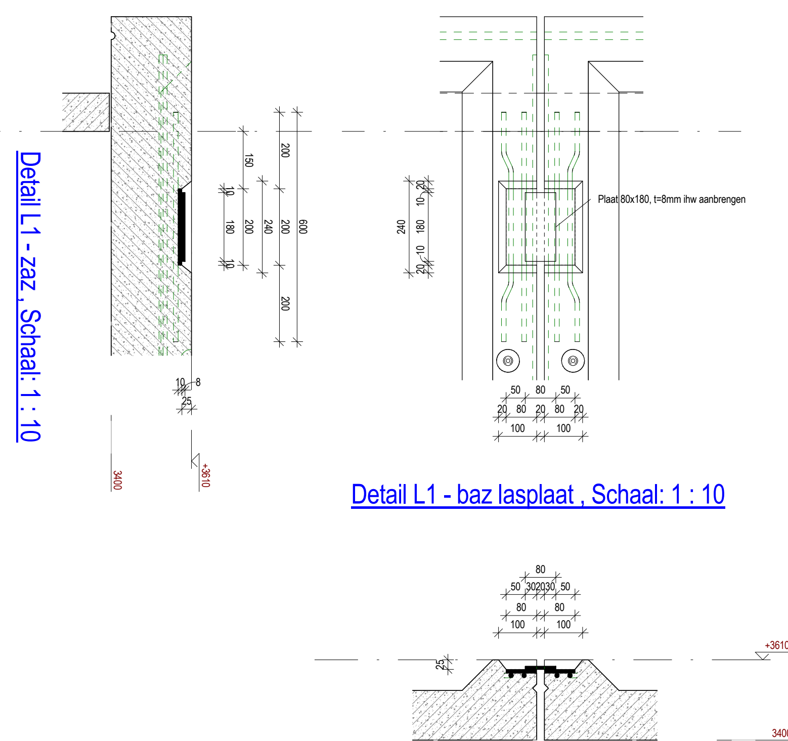
Detail L1 - dsn, Schaal: 1 : 10
