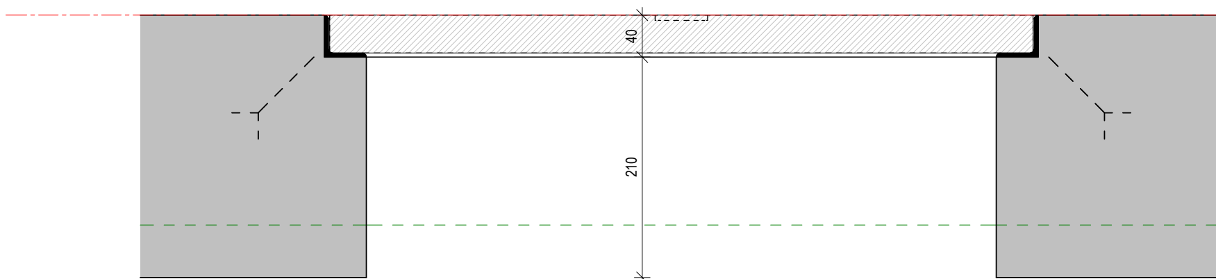
Detail Vloerluc , Schaal: 1 : 5
