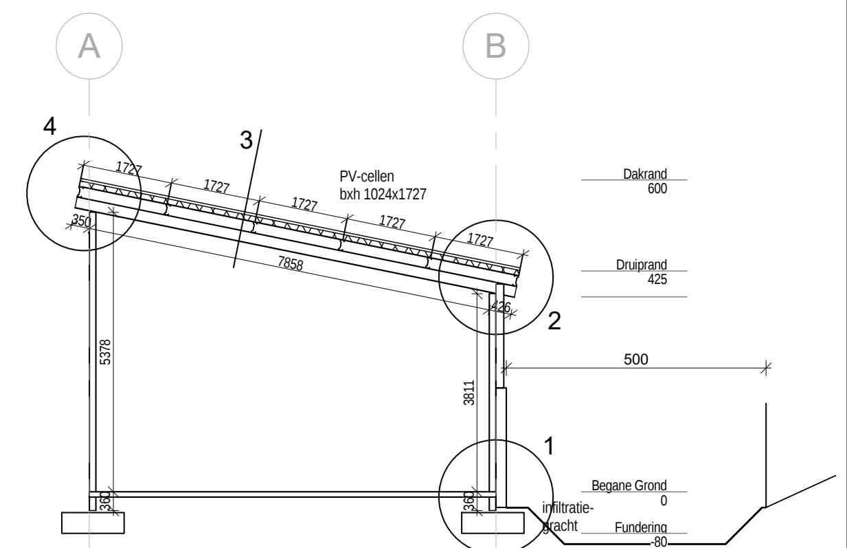
Doorsnede A
