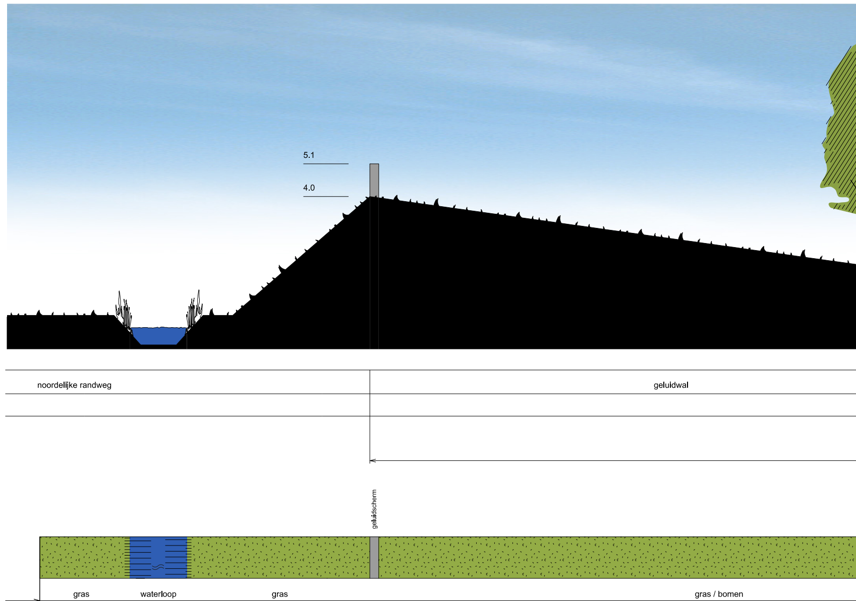
PROFIEL E
