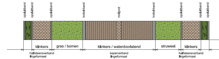
PROFIEL C
