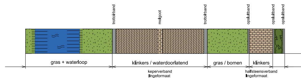
PROFIEL B-B
