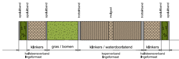
PROFIEL C-C
