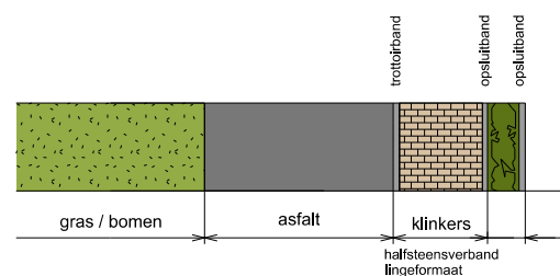
PROFIEL D
