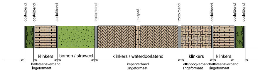
PROFIEL B
