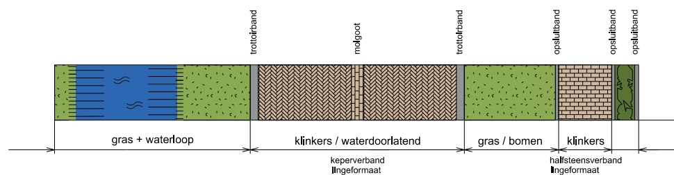
PROFIEL B-B
