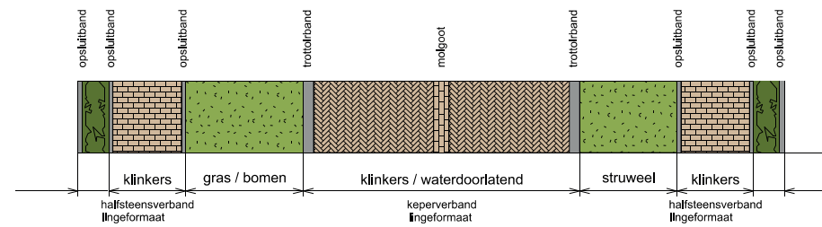
PROFIEL C
