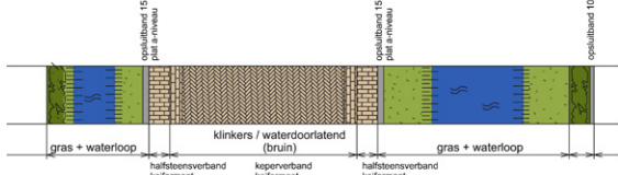
PROFIEL 2 / ST. DONATUSKAPTELSTRAAT
