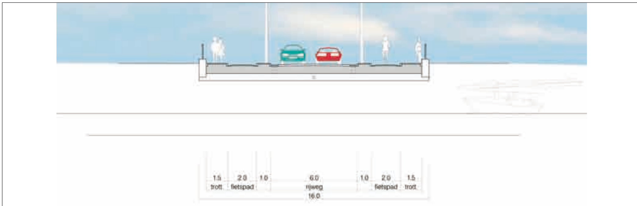
Profiel verkeersbrug
