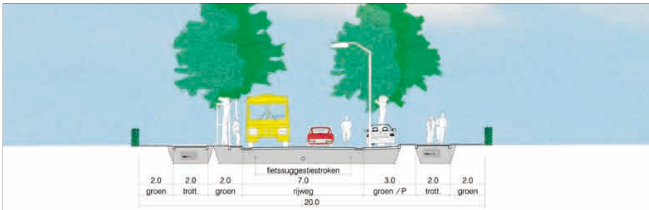
Profiel wijkontsluitingsweg
