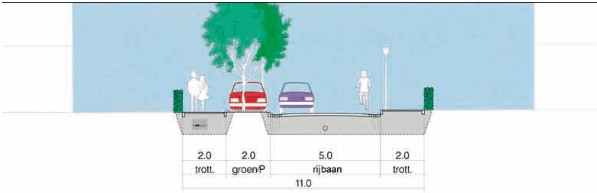
Profiel woonstraat
