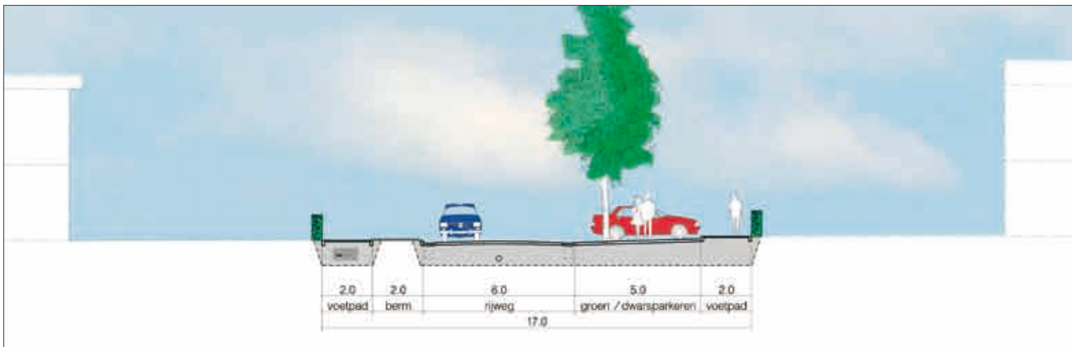
Profiel buurtontsluitingsweg
