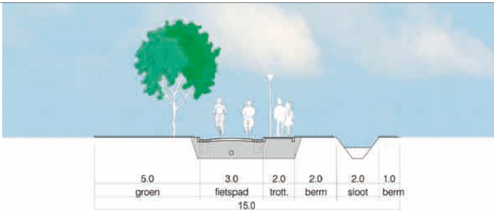
Profiel langzaamverkeerroute
