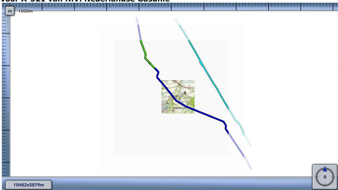
Figuur 4.2 Kilometer leiding behorende bij de maximale overschrijding van de FN-curve voor A-521 van N.V. Nederlandse Gasunie
