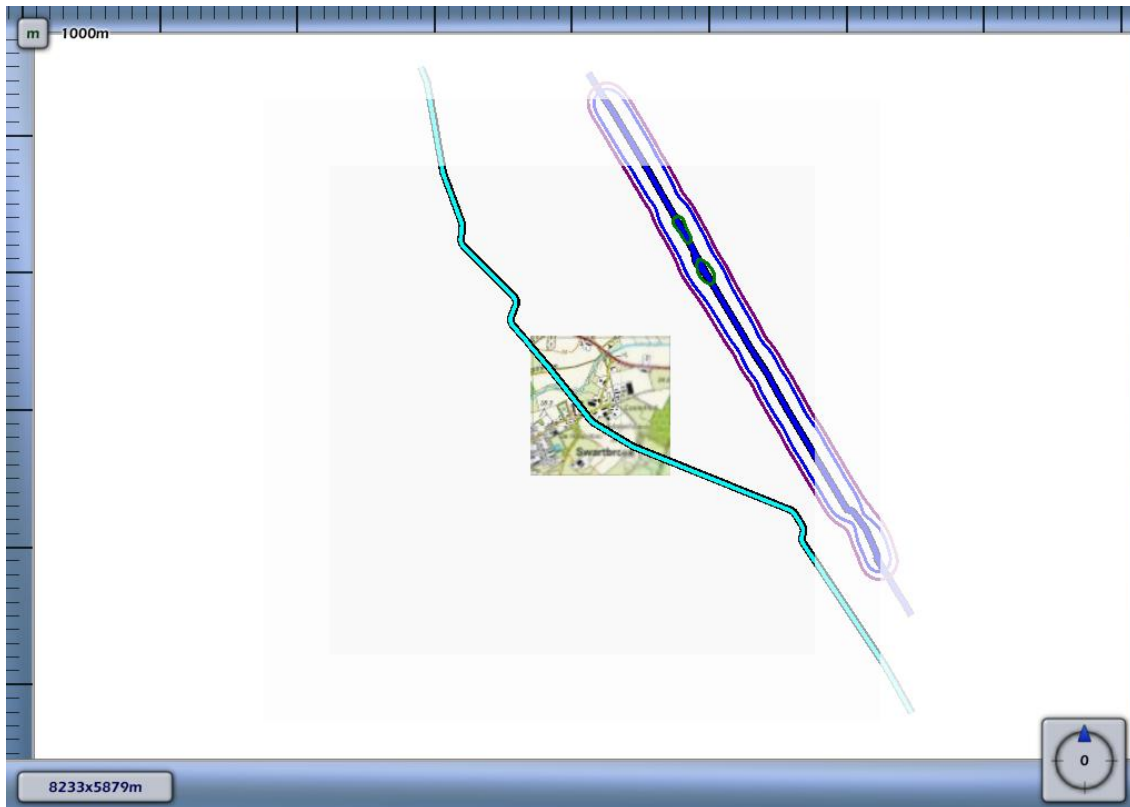
3.1 Figuur 3.1 Plaatsgebonden risico voor Z-540-01 van N.V. Nederlandse Gasunie
