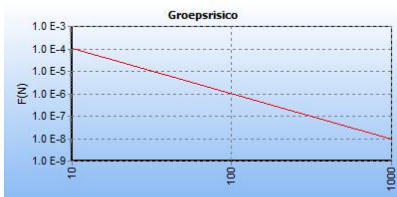
5.3 Figuur 5.3 FN curve voor A-585 van N.V. Nederlandse Gasunie voor de kilometer tussen stationing 50470.00 en stationing 51470.00
