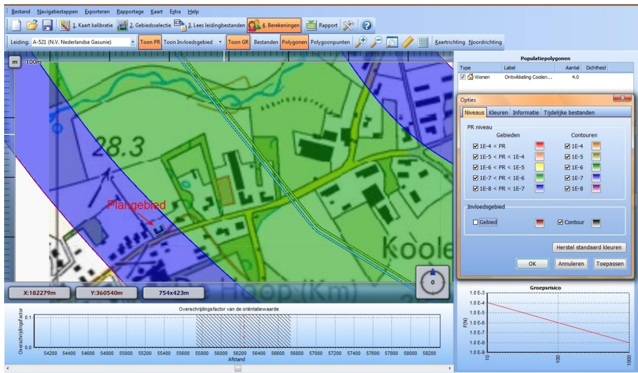
Plaatsgebonden risicocontouren buisleiding A-521 en ligging plangebied
